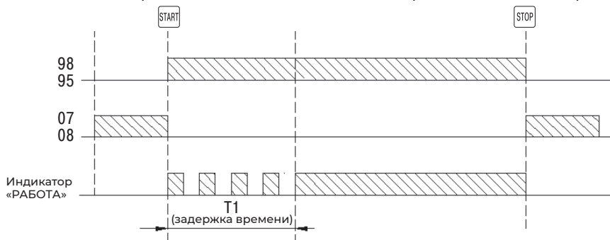
Рис. 14. Схема последовательности запуска
