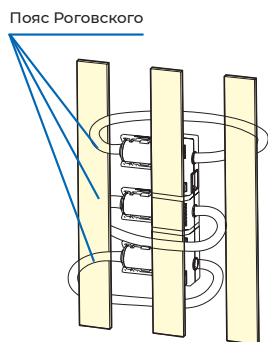
Рис. 5. Вариант 1 установки трансформатора с поясом Роговского
