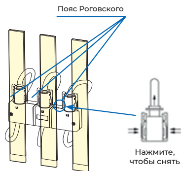
Рис. 6. Вариант 2 установки трансформатора с поясом Роговского
