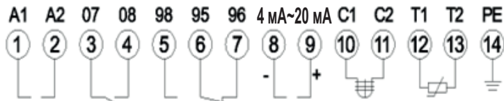
Рис. 9. Обозначения контактов
