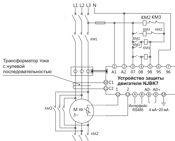
Рис. 12. Схема соединений, запуск «звезда/треугольник»
