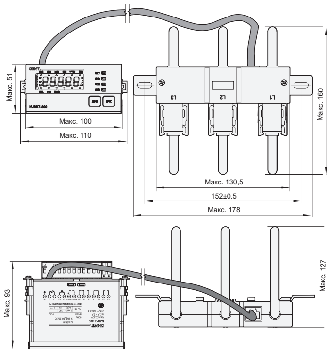
Рис. 4. Габаритные и установочные размеры устройства защиты с номинальным током 400, 800 А
