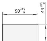
Рис. 7. Размеры монтажного отверстия для блока управления
