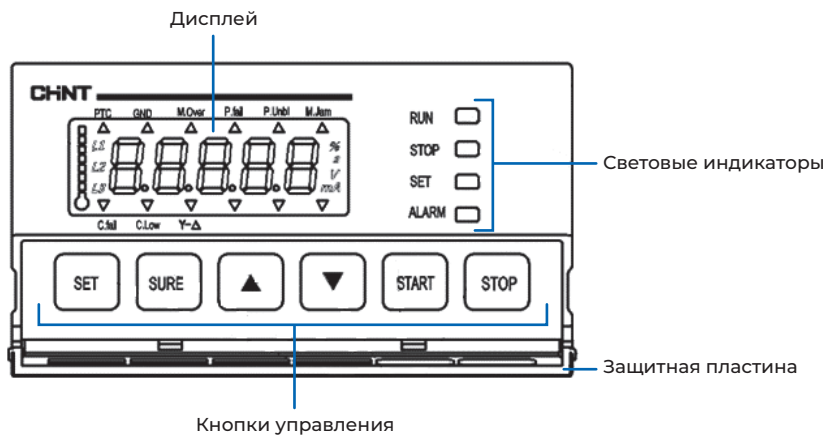
Рис. 8. Схема панели
