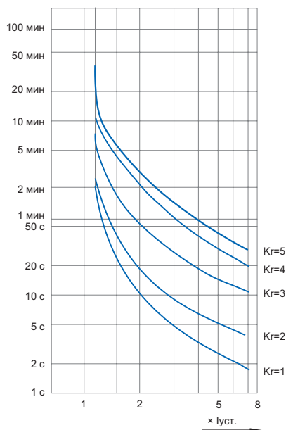
Рис. 1. Время-токовая характеристика
