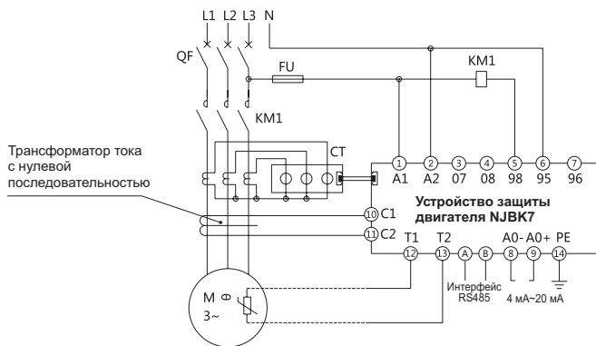
Рис. 11. Схема соединений, прямой запуск с вспомогательной цепью
