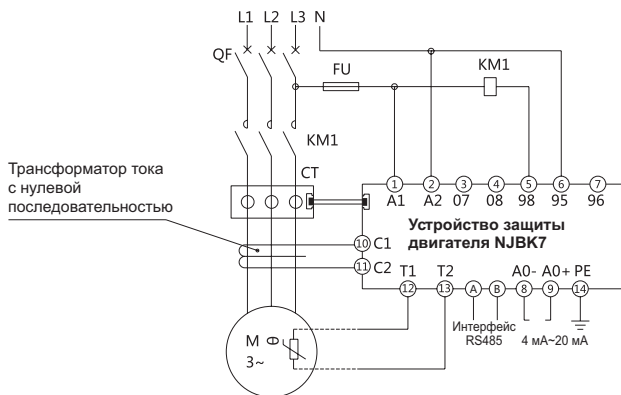
Рис. 10. Схема соединений, прямой запуск
