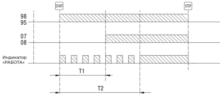
Рис. 15. Схема последовательности запуска
