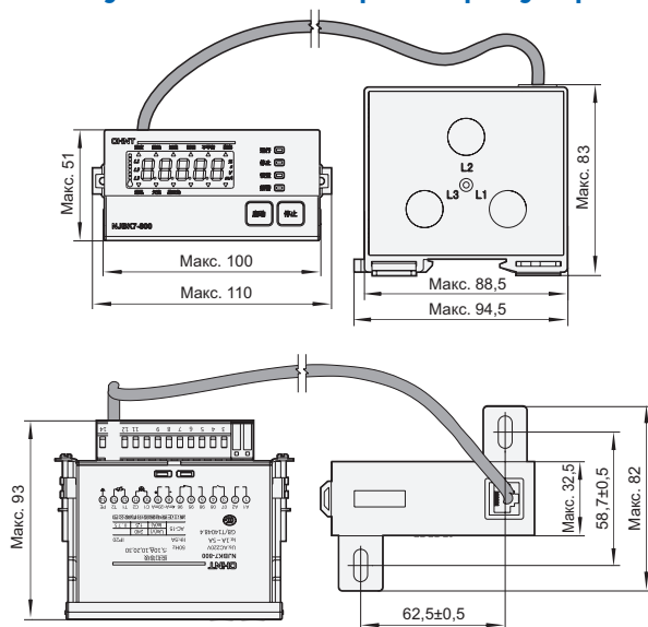
Рис. 2. Габаритные и установочные размеры устройства защиты с номинальным током 5, 10, 40 А
