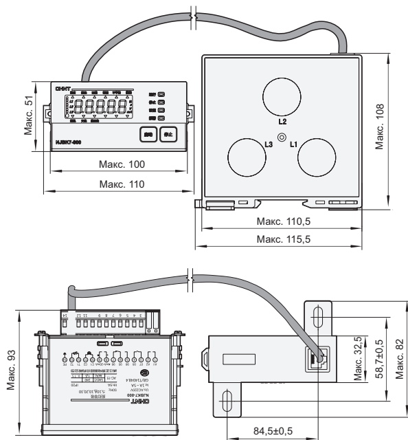
Рис. 3. Габаритные и установочные размеры устройства защиты с номинальным током 100 А
