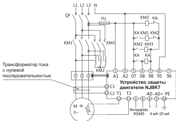
Рис. 13. Схема соединений, запуск самокоммутиацией
